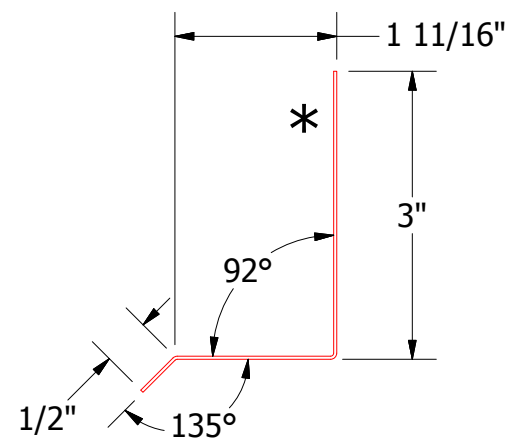
MDA660-Plain Sill Trim
